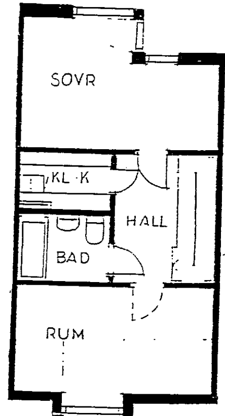
ÖVRE PLAN
