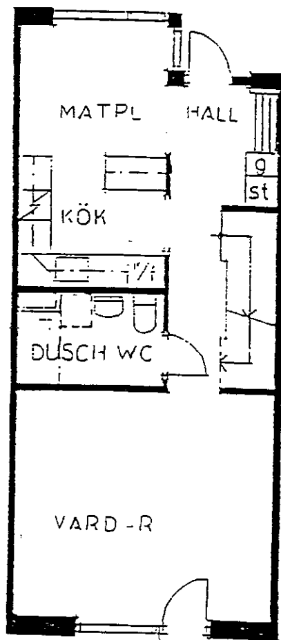
NEDRE PLAN
